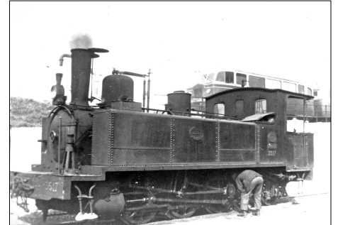
847 CF – BOURGES (18) Locomotive SACM 031 T n° 3517 au dépôt. © Maurice RIFAULT - 1946.
