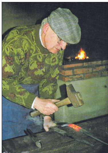
Fabrication du bochard Louis BOUCHET Charron à Villefort met en forme sur l'enclume un bichard. Février 1999 Photo Jean-Louis Maurin N°39 Éditions Quand le passé laisse un message
